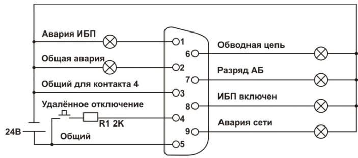
Рисунок 14 – Электрическая схема организации контроля и управления ИБП с электропитанием от источника постоянного тока напряжением +24 В
