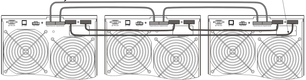
Рисунок 29 – Подключение информационных кабелей к трем ИБП в параллельной системе
