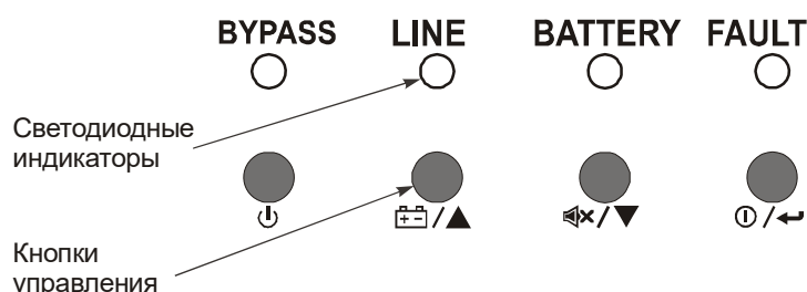
Рисунок 2 – Внешний вид органов управления и индикации ИБП
