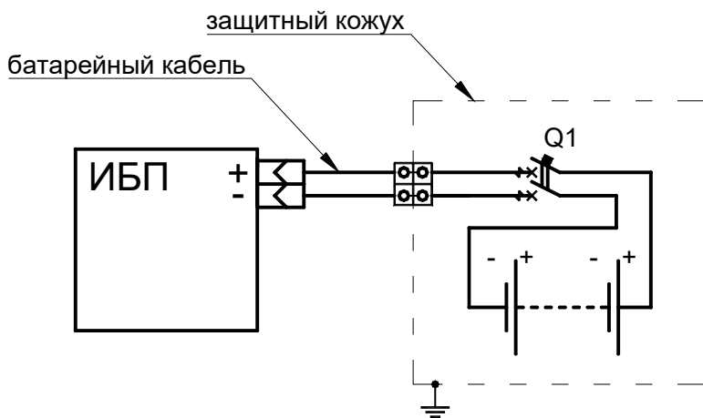
Рисунок 12 – Схема электрическая подключения аккумуляторов к ИБП
